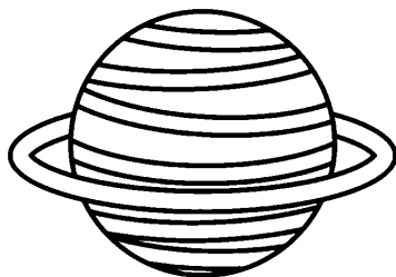
URANUS
