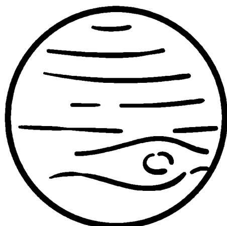
Jupiter
