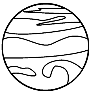
VENUS
