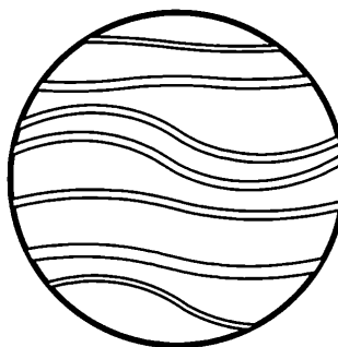
JUPITER
