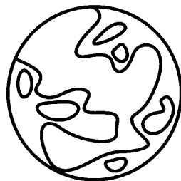
MARS
