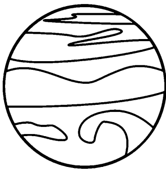
VENUS
