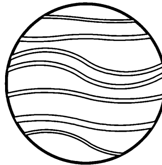
JUPITER
