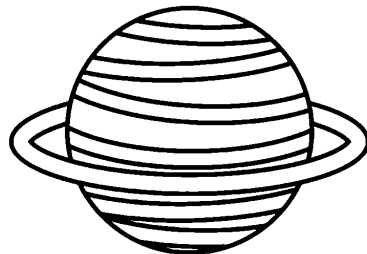
URANUS
