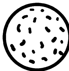
Mars
